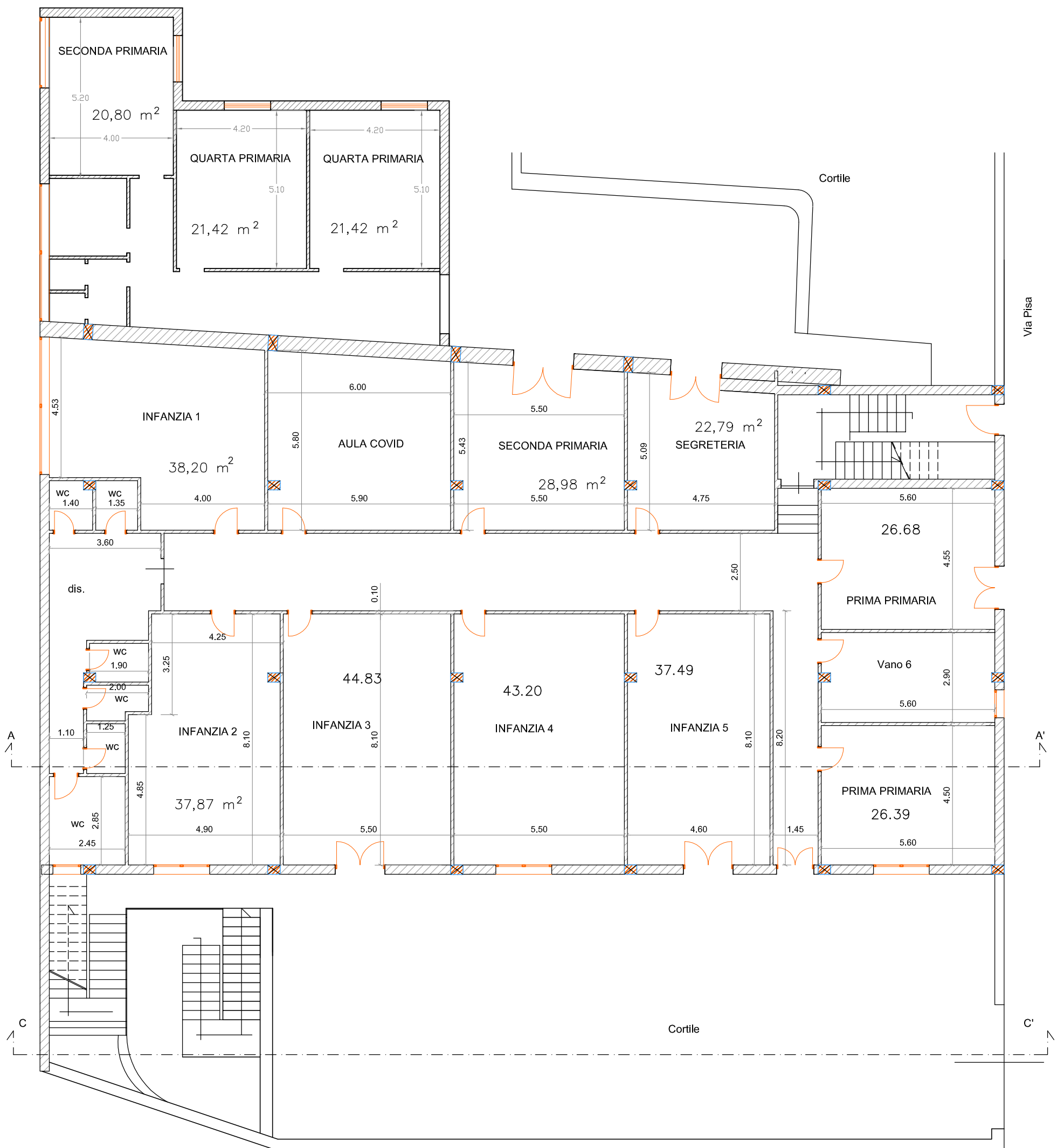
N Pianta piano terra di progetto scala 1:100
